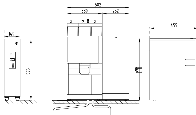
Voorzijde
