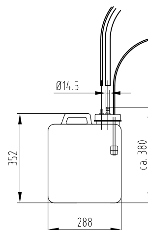
Vuil-water tank 13L
