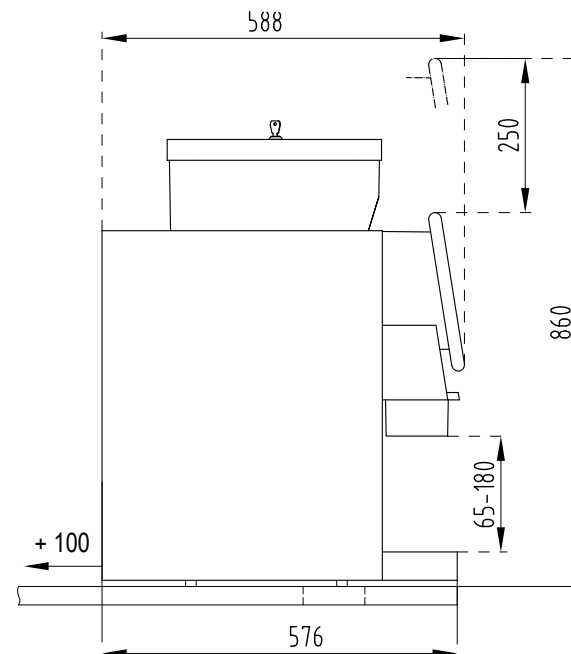
Zij-aanzicht machine
