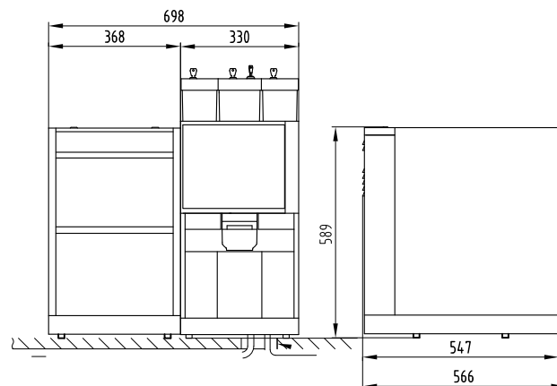
Voorzijde
