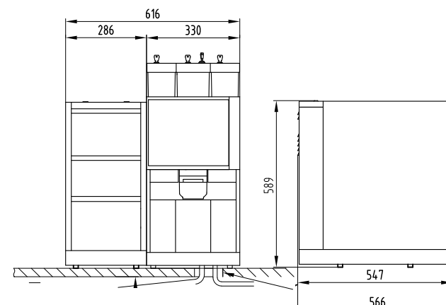
Voorzijde
