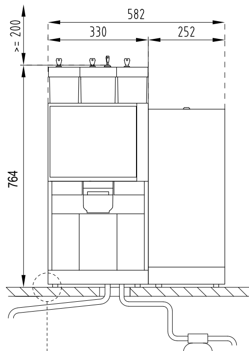
Voorzijde machine
