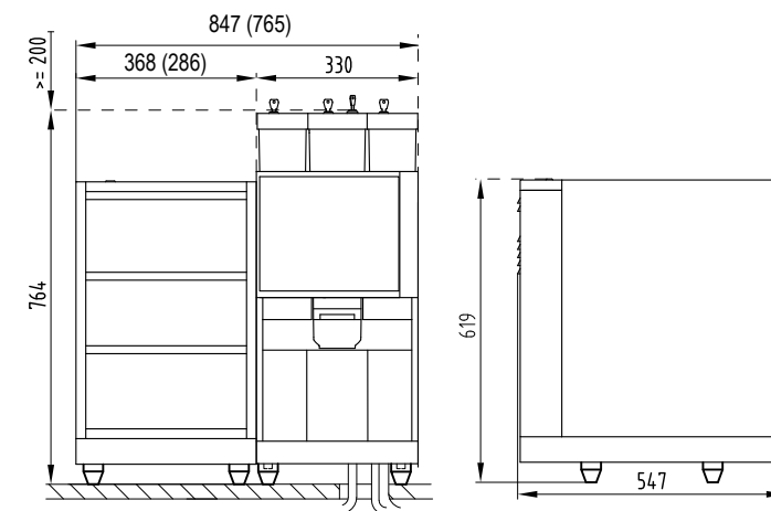
Voorzijde
