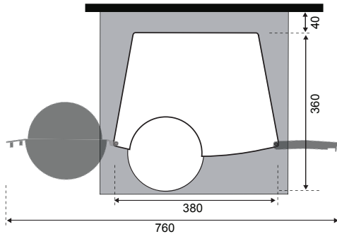
Bovenaanzicht (met geopende deuren)
